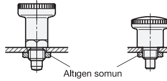
GN 607 / GN 607.1 indeksleme pistonları
