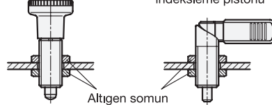
GN 612 kam hareketi indeksleme pistonu
